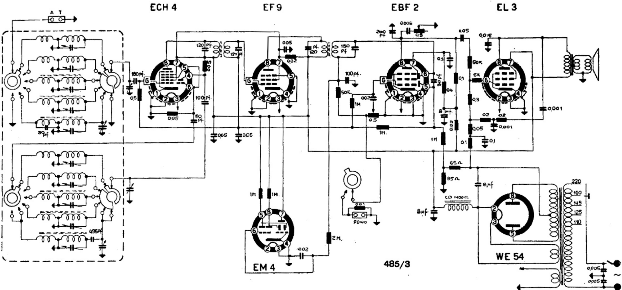
MINERVA RADIO - Mod. 485.3 « PASUBIO » e mod. 1485.3 « BERNINA » - Gamma medie da 200 a 580 m, corte da 36,5 a 52 m e da 27 a 38 m, cortissime da 19 a 27,5 m e da 13,5 a 19,5 m. Media frequenza 470 kc/s. Potenza d'uscita 4 W. Consumo 65 W.
